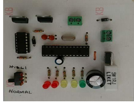
Şekil 2. 36 V iki seviyeli akü şarj devresi
