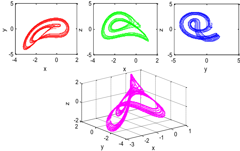
Şekil 1. GRSÜ üretimde kullanılan kaotik sistemin faz görünümü.
